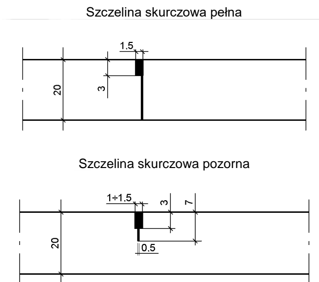
Rys. 1.1. Przykłady konstrukcji szczelin w podbudowie z betonu cementowego (wymiarów w cm)
